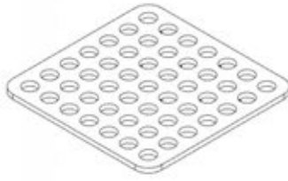
S01 ECRAN - A4M02005 (x4) 1/16"x2 11/16"x2 11/16" (2x68x68)
