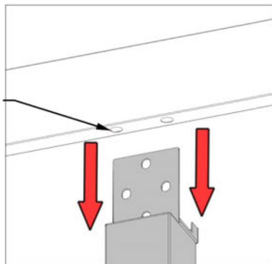
VUE ARRIÈRE
