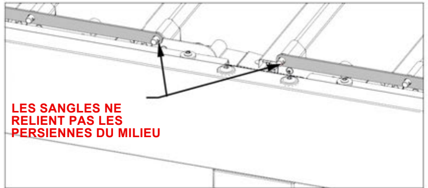
F02 SANGLE DE LIAISON À PERSIENNE -A4M02586 (x4) 1/8"x5/8"x108 3/8" (3x16x2752)
