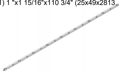
M01 BÂTI À PERSIENNES - A4M02596 (x1) 1 "x1 15/16"x110 3/4" (25x49x2813)
