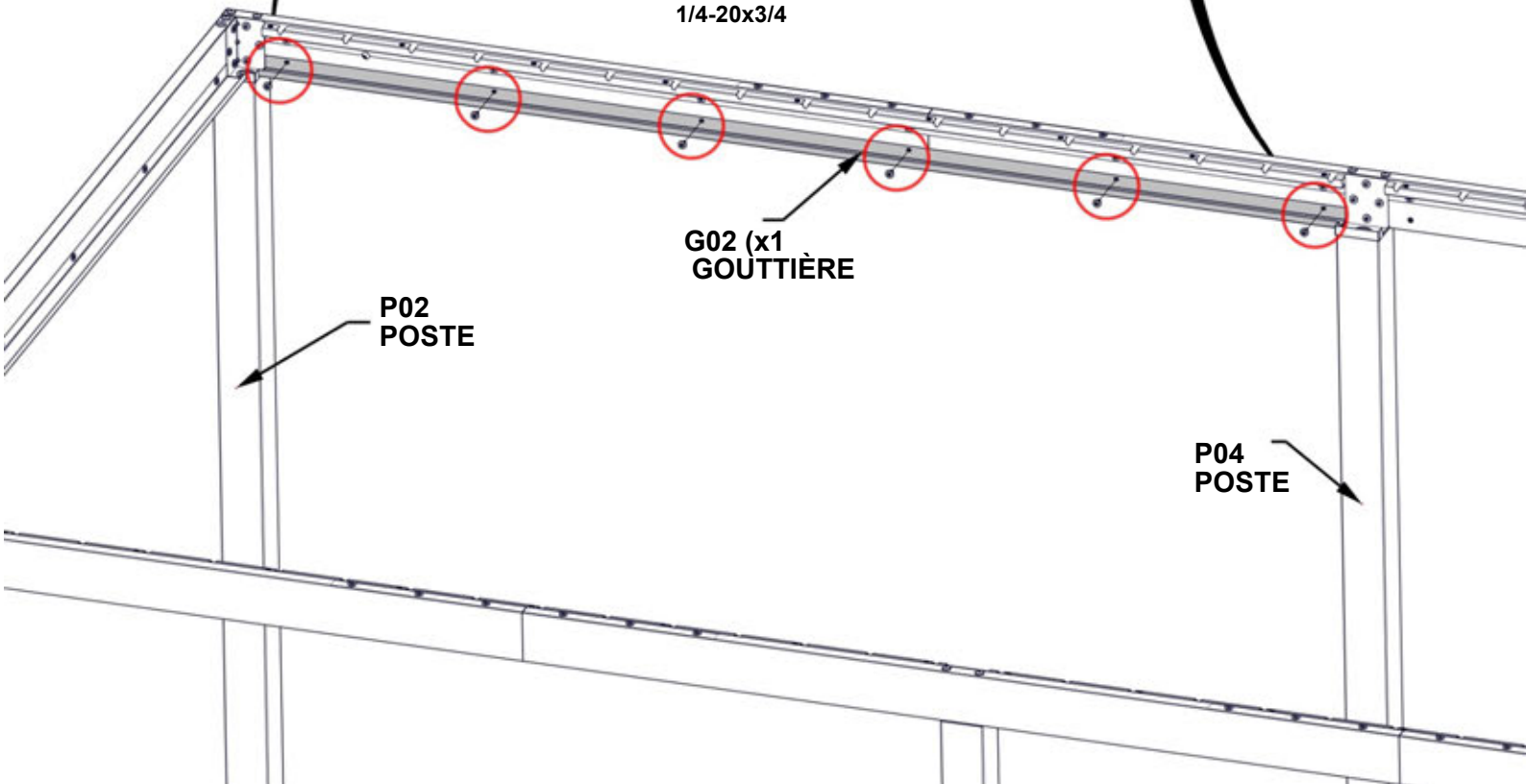
1202 (x6) ENSEMBLE TÊTE PORTE- PLATEAU TORX 1/4-20x3/4
