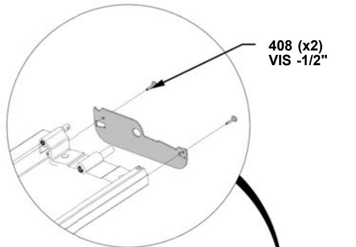
L03 (x1) PLAQUE LATÉRALE DE PERSIENNE
