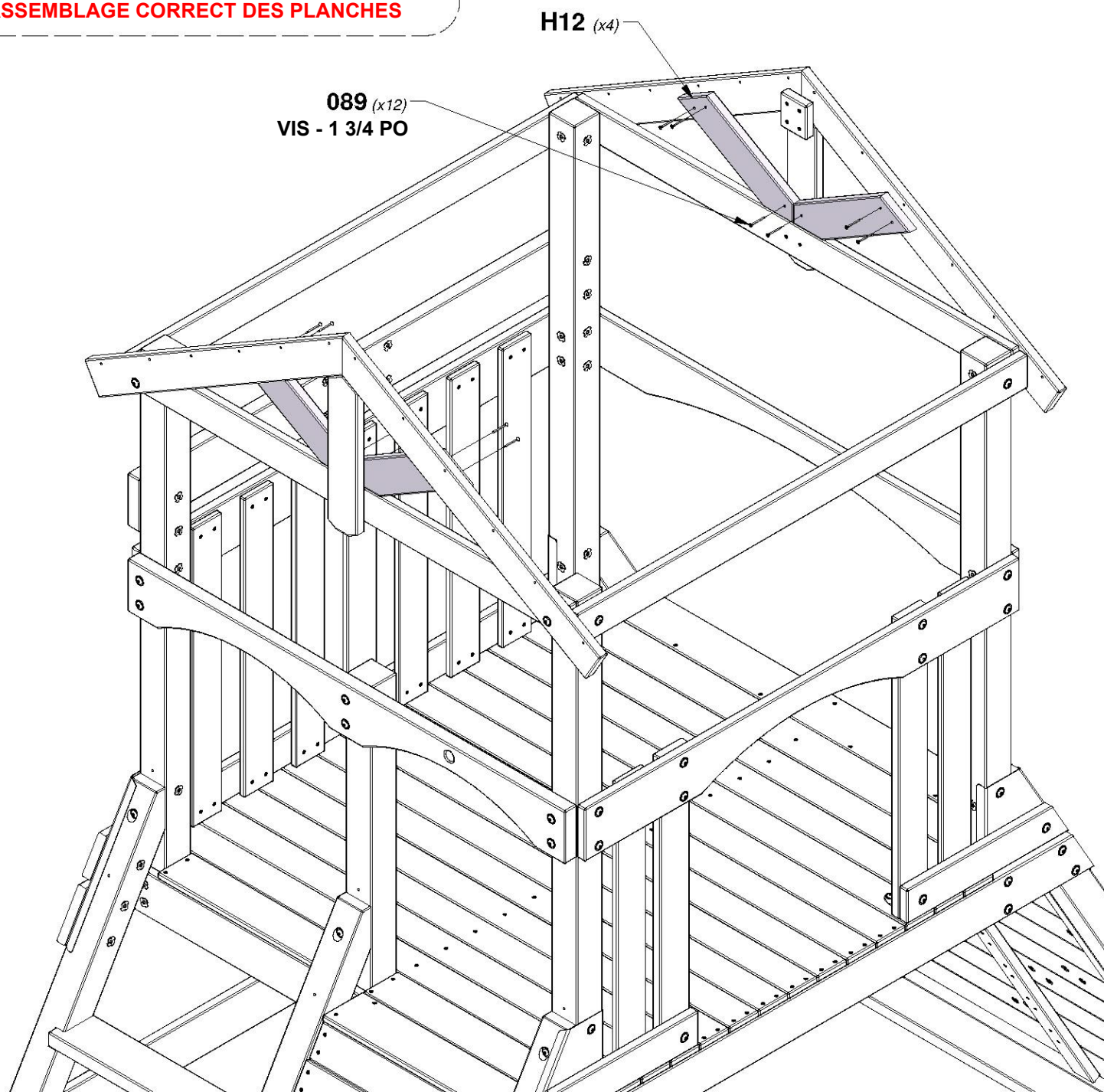
ASSEMBLAGE CORRECT DES PLANCHES
