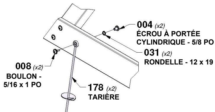
DÉTAIL - « A »
