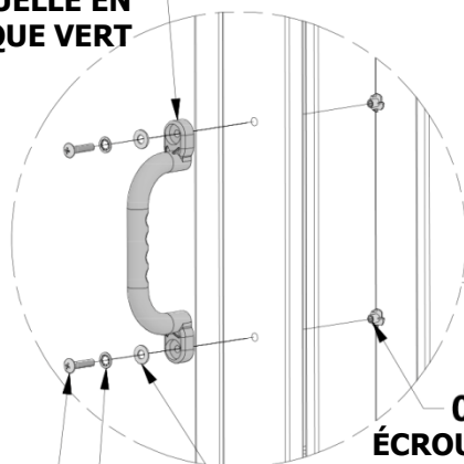
106 (x4) RONDELLE - 9x18
