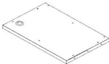
T2 ASSEMBLAGE DU DESSUS DE TABLE - A4M05455 (x1) 38 1/4 po x 25 po x 1 9/16 po (40 x 635 x 971)
