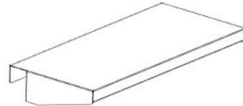
A7 ÉTAGÈRE ARRIÈRE - A4M06229 (x4) 2 7/16 po x 7 15/16 po x 17 11/16 po (61 x 201 x 450)
