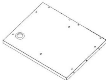
T4 ASSEMBLAGE DU DESSUS DE TABLE - A4M05470 (x1) 31 7/16 po x 25 po x 1 9/16 po (40 x 635 x 798)
