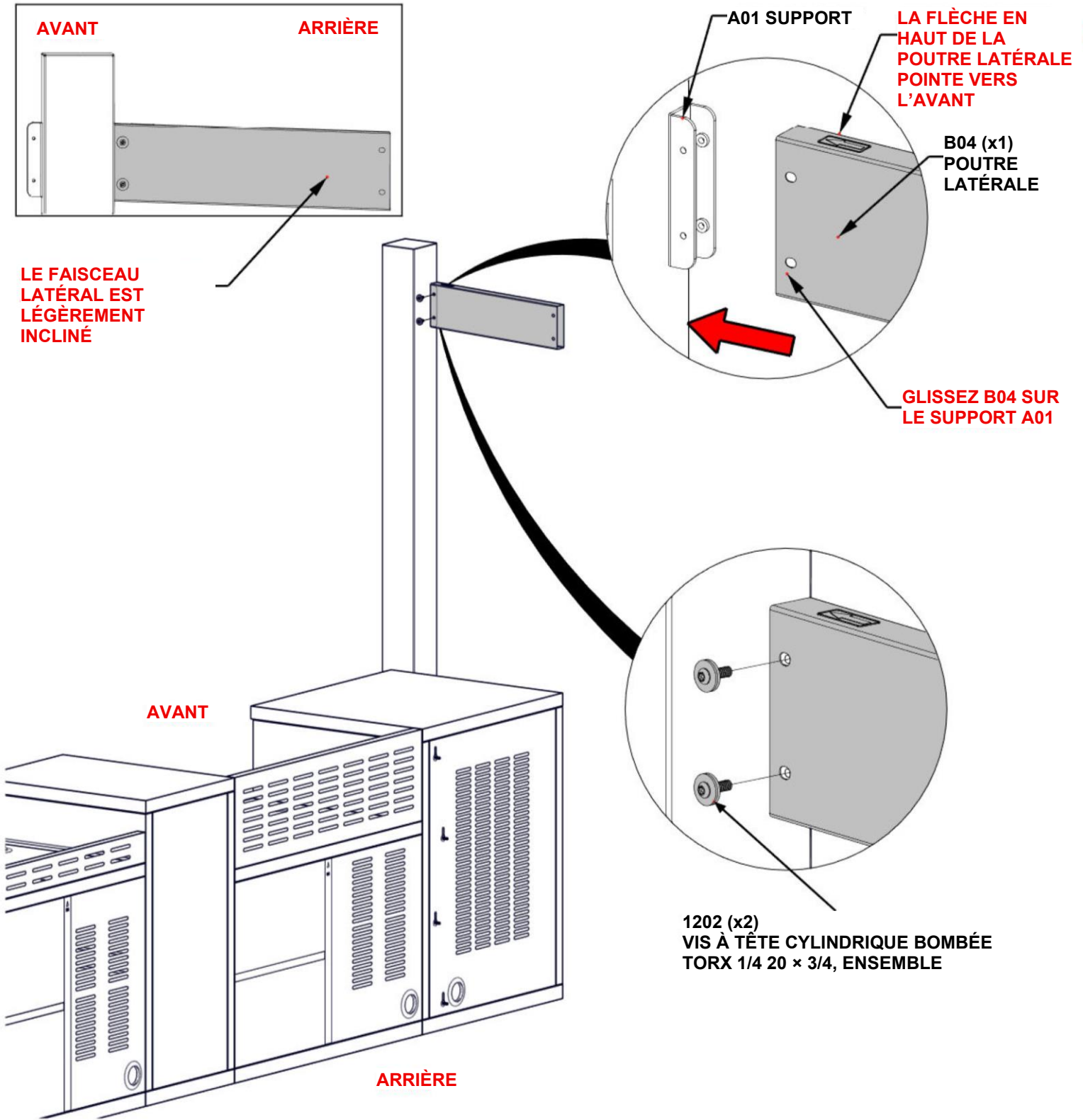
B04 POUTRE LATÉRALE - A4M02019 (x1) 1 7/16 po x 5 1/4 po x 18 7/8 po (36 x 134 x 480)
