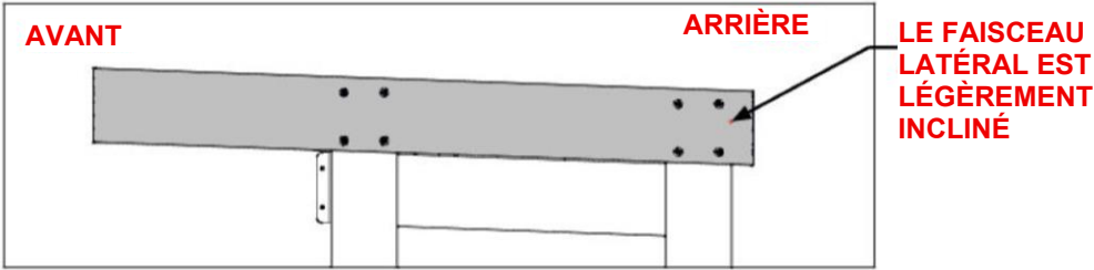
B05 POUTRE LATÉRALE - A4M02022 (x1) 1 7/16 po x 5 1/4 po x 46 1/2 po (36 x 134 x 1181)
