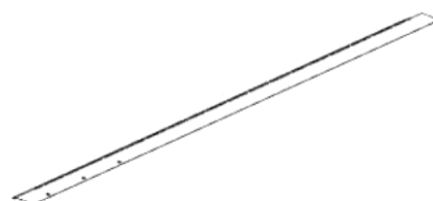
5506 (x1) BORD D'ÉGOUTTEMENT - A4M05506 3/16 po x 3 7/16 po x 78 1/4 po (6 x 88 x 1987)
