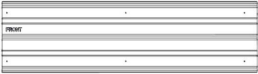
5500 TÔLE D'ACIER 29GA - A4M05500 (x1) 1/4 po x 13 po x 46 7/16 po (7 x 330 x 1179)
