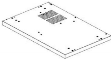
F8 ASSEMBLAGE DU PANNEAU DE PLANCHER - A4M05758 (x1) 38 1/4 po x 25 po x 1 3/4 po (45 x 635 x 971)
