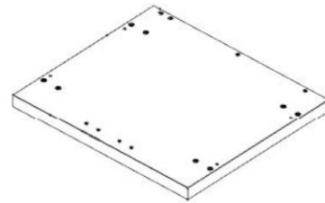
F5 ASSEMBLAGE DU PANNEAU DE PLANCHER - A4M05473 (x1) 28 5/8 po x 25 po x 1 3/4 po (45 x 635 x 727)
