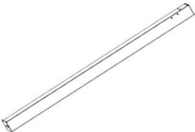
P01 ASSEMBLAGE DU MONTANT AVANT - A4M05508 (x1) 4 3/4 po x 5 15/16 po x 89 1/2 po (120 x 151 x 2274)
