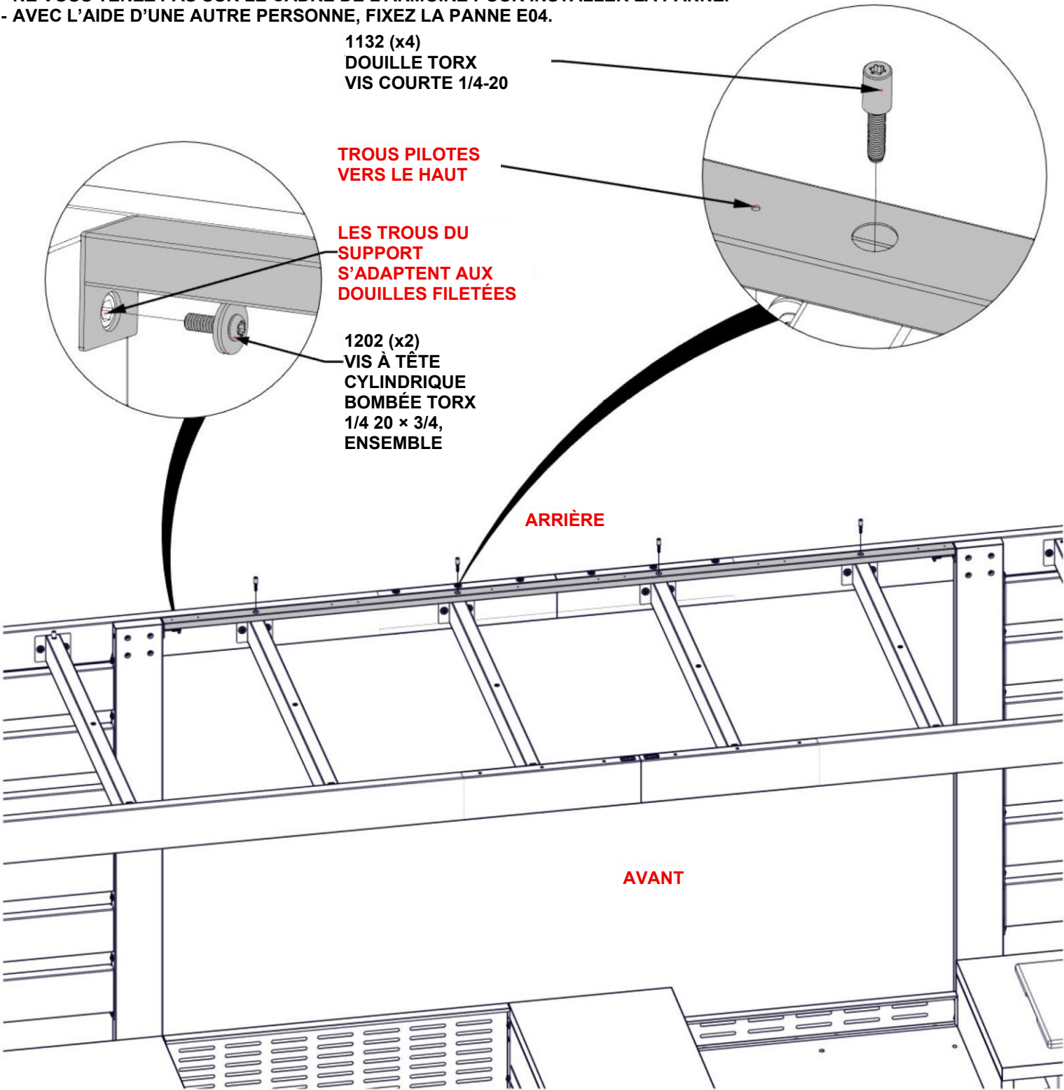
E04 ASSEMBLAGE DE LA PANNE - A4M05501 (x1) 1 9/16 po x 1 3/4 po x 87 13/16 po (40 x 45 x 2230)
