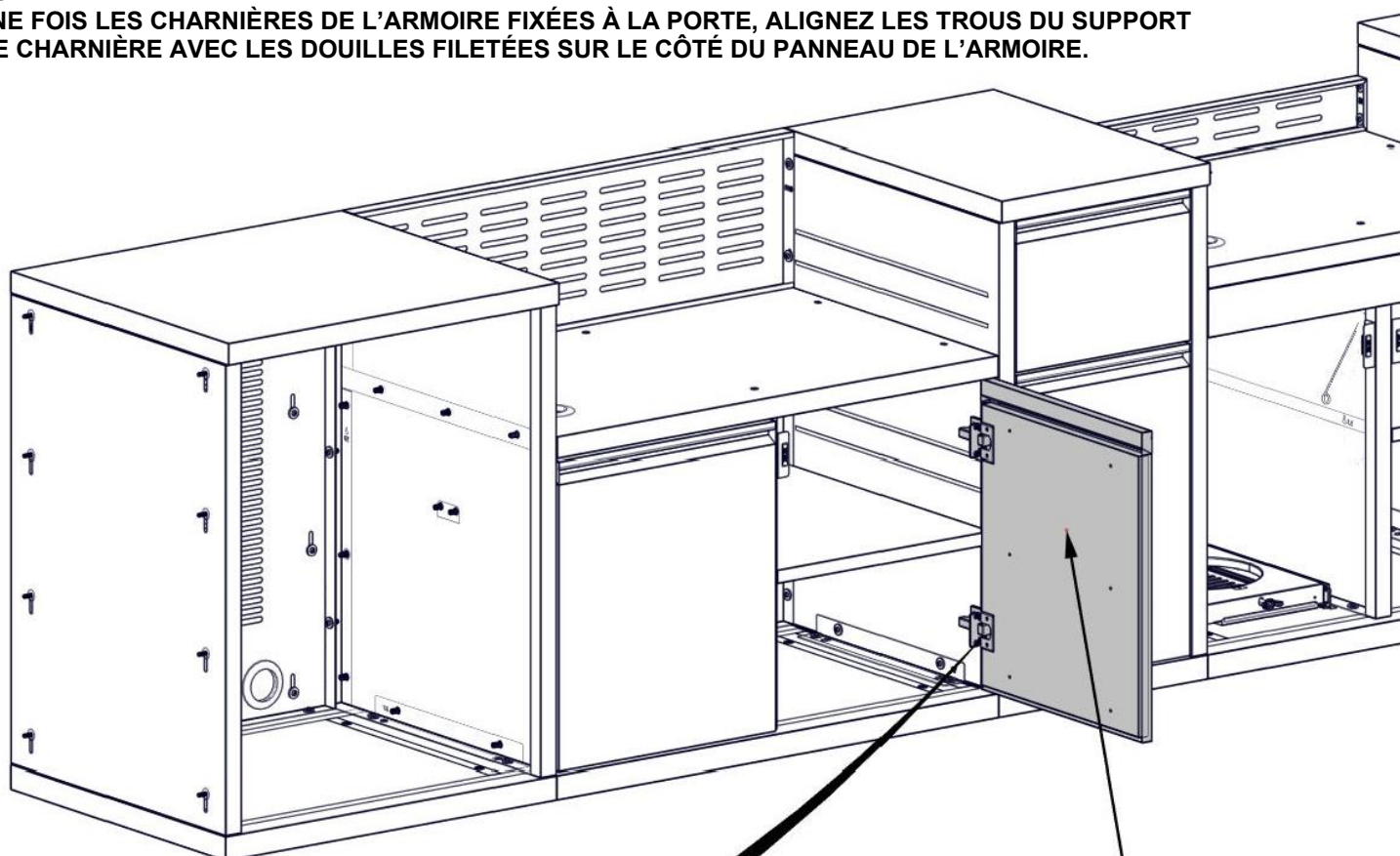
D1 (x1) ASSEMBLAGE DE PORTE
