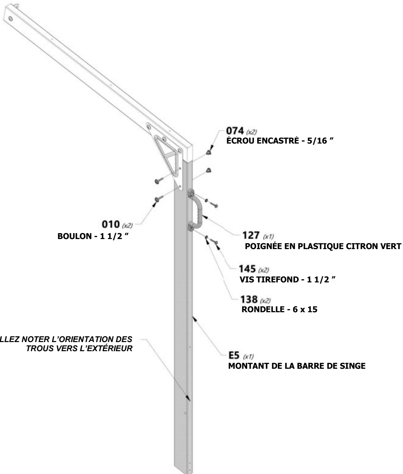
A6P00127 | POIGNÉE EN PLASTIQUE (1) | CITRON VERT
