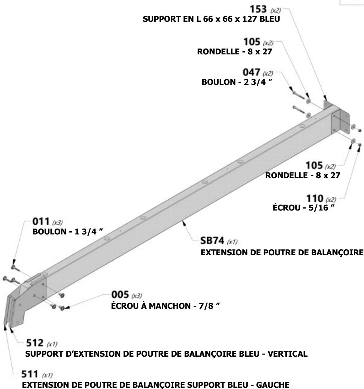
A4M00511 (1) EXTENSION DE POUTRE DE BALANÇOIRE SUPPORT BLEU - GAUCHE
