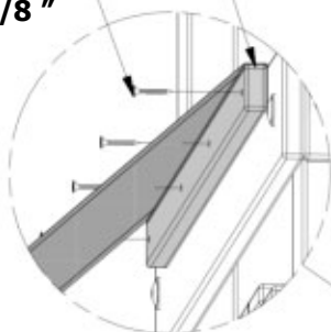
088 (x4) VIS - 1 1/8 "
