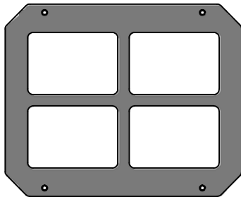
(3) GK - FENETRE 216x267 VERTE - A100146
