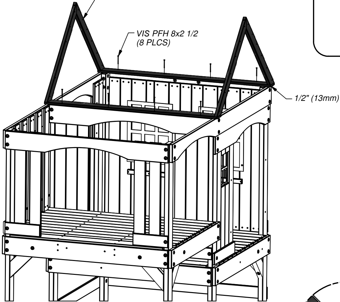
MONTAGE DE LA BASE DU TOIT
