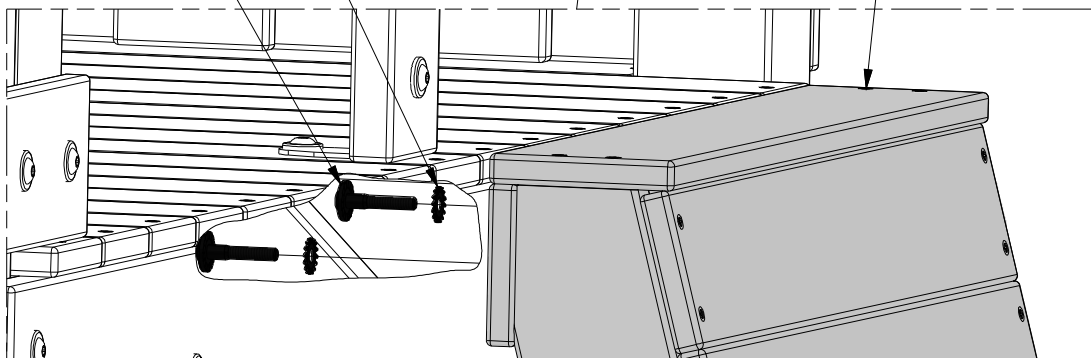
407 (x2) BOLT - 1 1/2"
