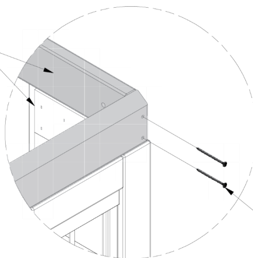
201 (x4) TORNILLO: 2 1/2"
