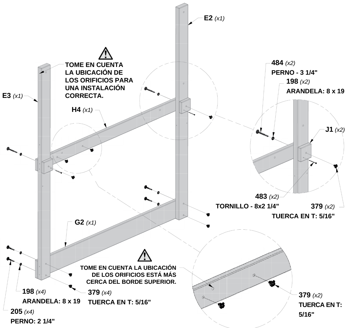
H100484 | PERNO BL NG (x2) | 5/16x3 1/4
