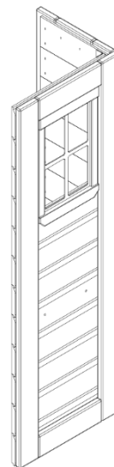
WP2 | PANEL DE ESQUINA TRASERO (x1) | DERECHO - W2A03154
