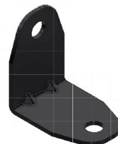
A4M01047 (x3) | SOPORTE EN ESCUADRA 2.5x38x55x55
