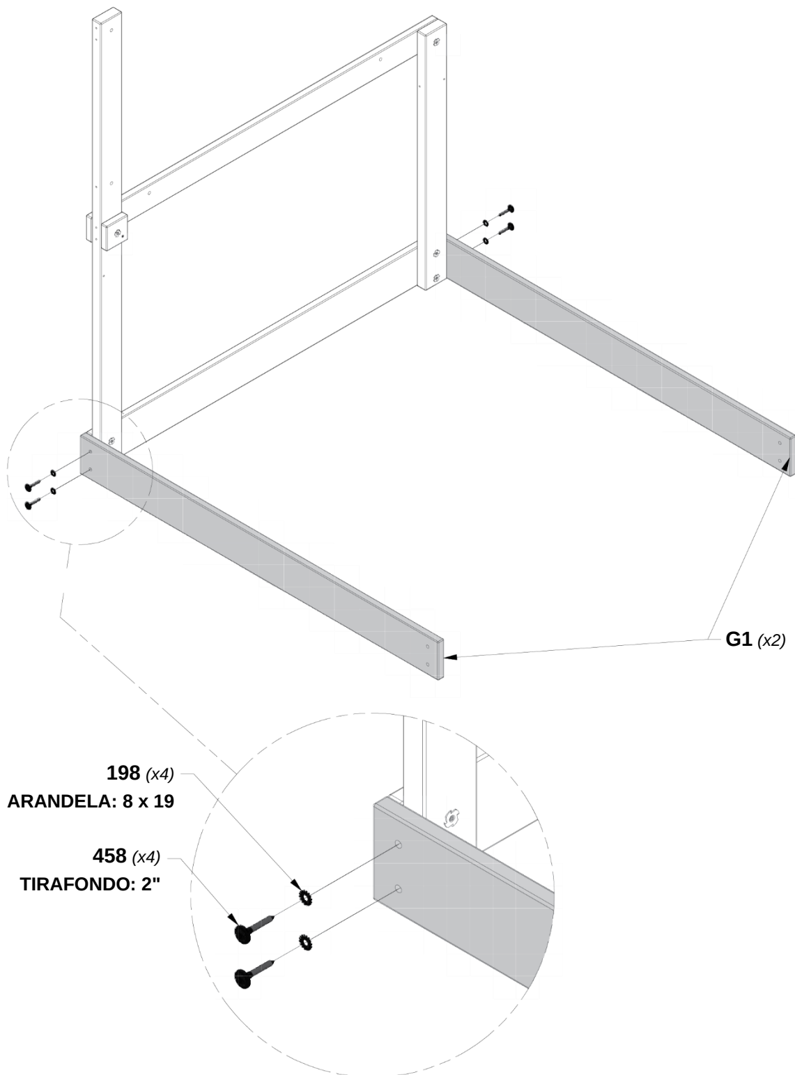
H100198 | ARANDELA DE (x4) | FIJACIÓN EXT. NG 8x19
