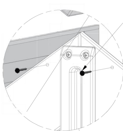
200 (x8) TORNILLO: 1 1/2"
