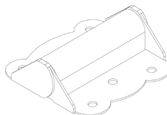
A4M00994 (x1) | BISAGRA (PUERTA, SIN RESORTE)
