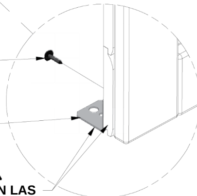
202 (x8) TORNILLO - 5/8"
