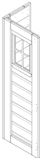
WP3 | PANEL DE ESQUINA DELANTERO (x1) | IZQUIERDO - W2A03157
