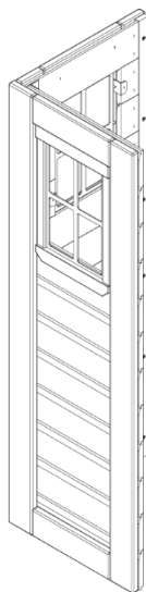
WP1 | PANEL DE ESQUINA DELANTERO (x1) | DERECHO - W2A03151
