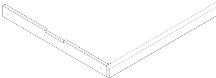
WP8 | CONJUNTO DE CABECERA - W2A03165 (x2)
