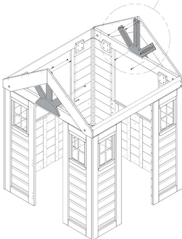
387 (x4) TORNILLO: 1 1/4"
