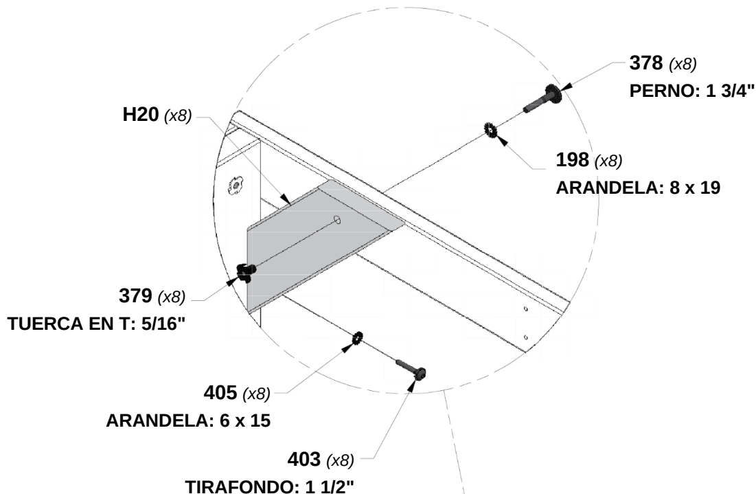
H20 | REFUERZO DE LA PLATAFORMA - (x8) | W4L14898 1 "x3 3/8" x13 "(24x86x330)
