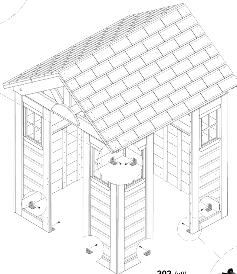
202 (x8) TORNILLO - 5/8"
