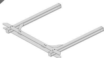
ASSEMBLAGE EN POSITION (x2) VERTICALE DES ÉTAPES PRÉCÉDENTES
