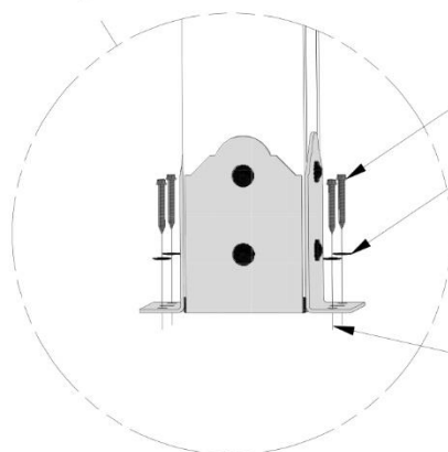
120 (x16) VIS - 2"
