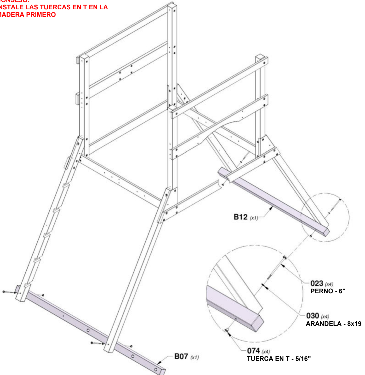
B07 | TABLA DEL SUELO - W4L15733 (x1) 3"x3"x89 3/8" (76x76x2270)
