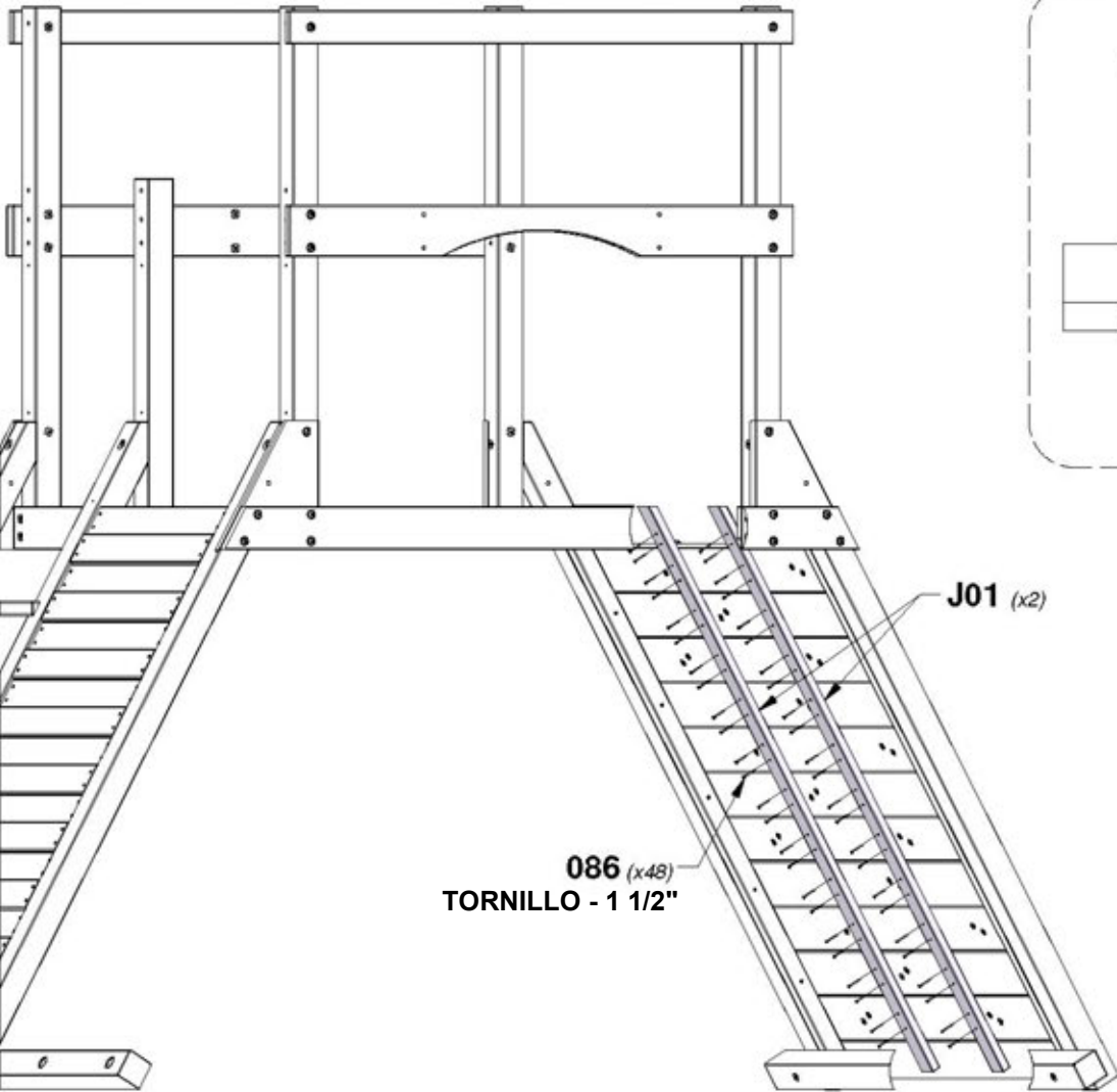
J01 | LISTÓN DEL MURO DE ESCALADA - W4L16447 (x2) 1"x2 3/8"x58 1/2" (24x60x1486)
