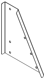
A4M01481 | A-FRAME BRACKET-RT (x2)
