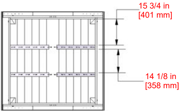
VISTA INFERIOR
