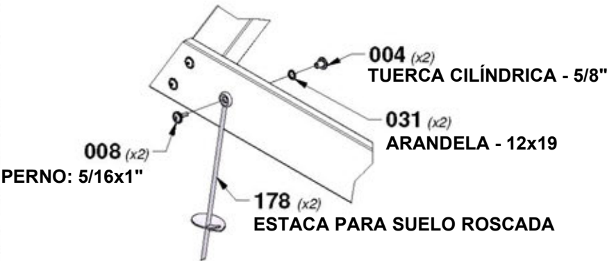
DETALLE - A
