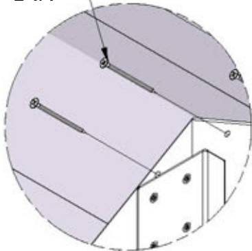
091 (x12) TORNILLO - 2 1/4"
