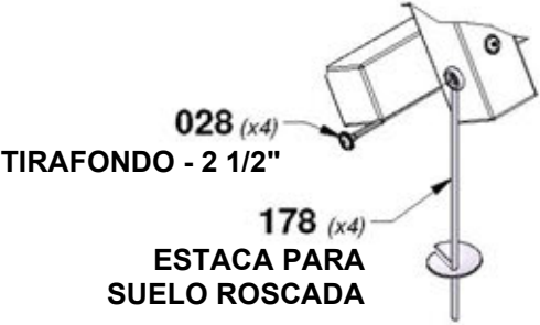
DETALLE - B
