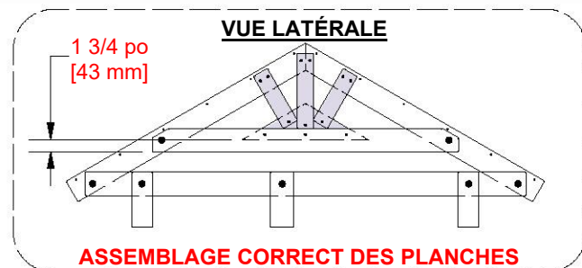
N02 ENCADREMENT DU PIGNON DE PORCHE AVANT - W4L16150 (x1) 5/8 po x 2 3/8 po x 10 7/8 po (16x60x275)
