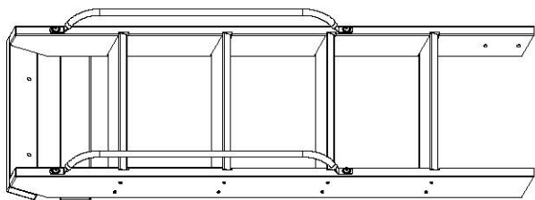
ASSEMBLAGE DE L'ÉCHELLE
