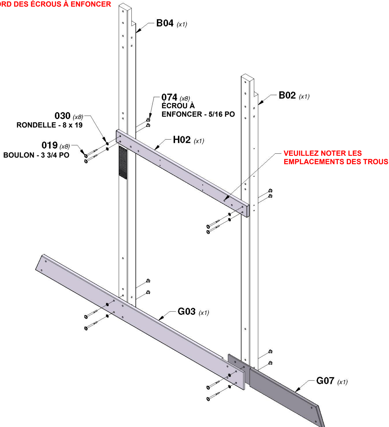
B04 MONTANT - W2A03406
