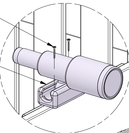
087 (x2) TORNILLO - 1-1/4"
