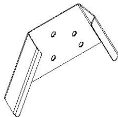
A4M01169 SOPORTE DE (x1) MARCO "A"
