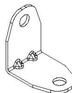
A4M01046 SOPORTE EN ESCUADRA (x2) 2.5x38x55x55
