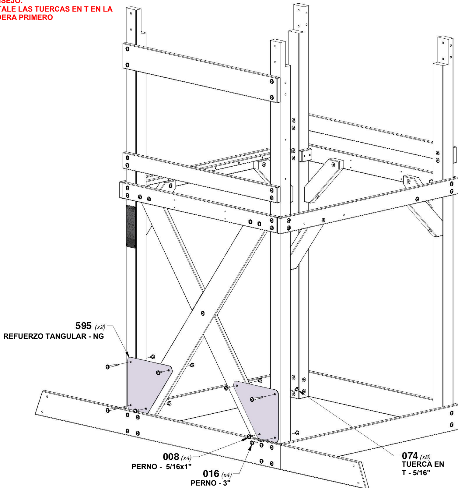
A4M01595 REFUERZO (x2) TANGULAR - NG
