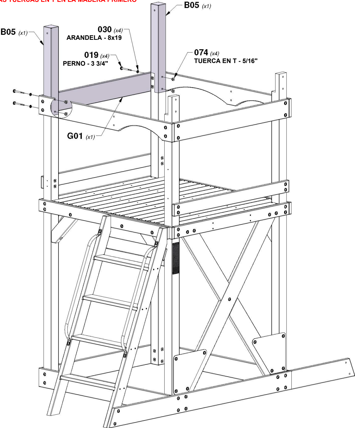
G01 GUÍA DEL SUELO - W4L16128 (x1) 1"x5 1/4"x44 7/8" (24x134x1141)
