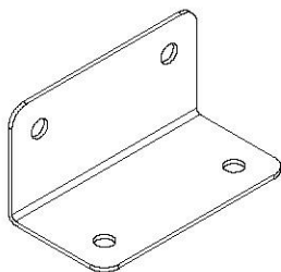
A100140 SOPORTE EN (x2) ESCUADRA 66x66x127
