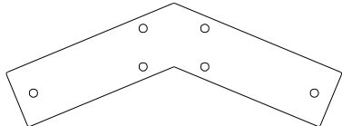
A4M01130 (x2) GABLE BRACKET
