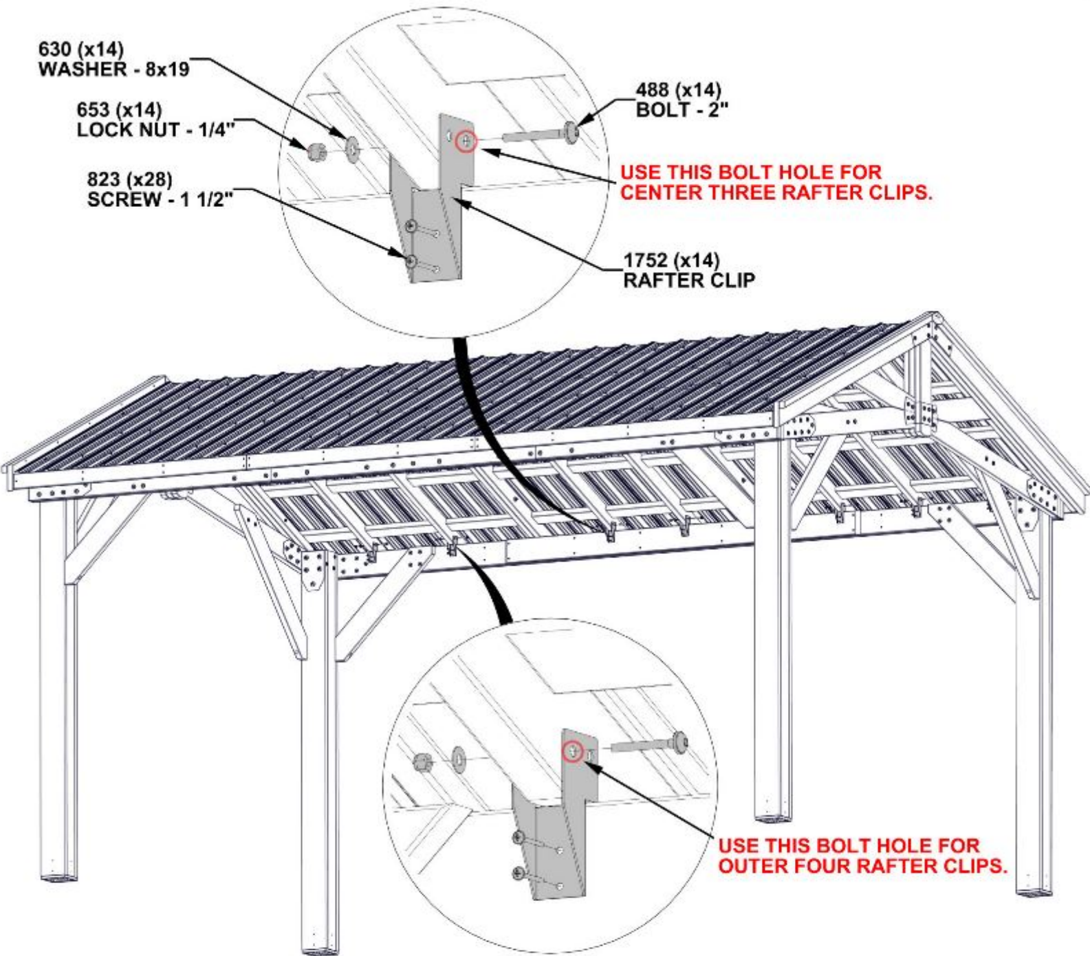
A4M01752 RAFTER CLIP (x14)
