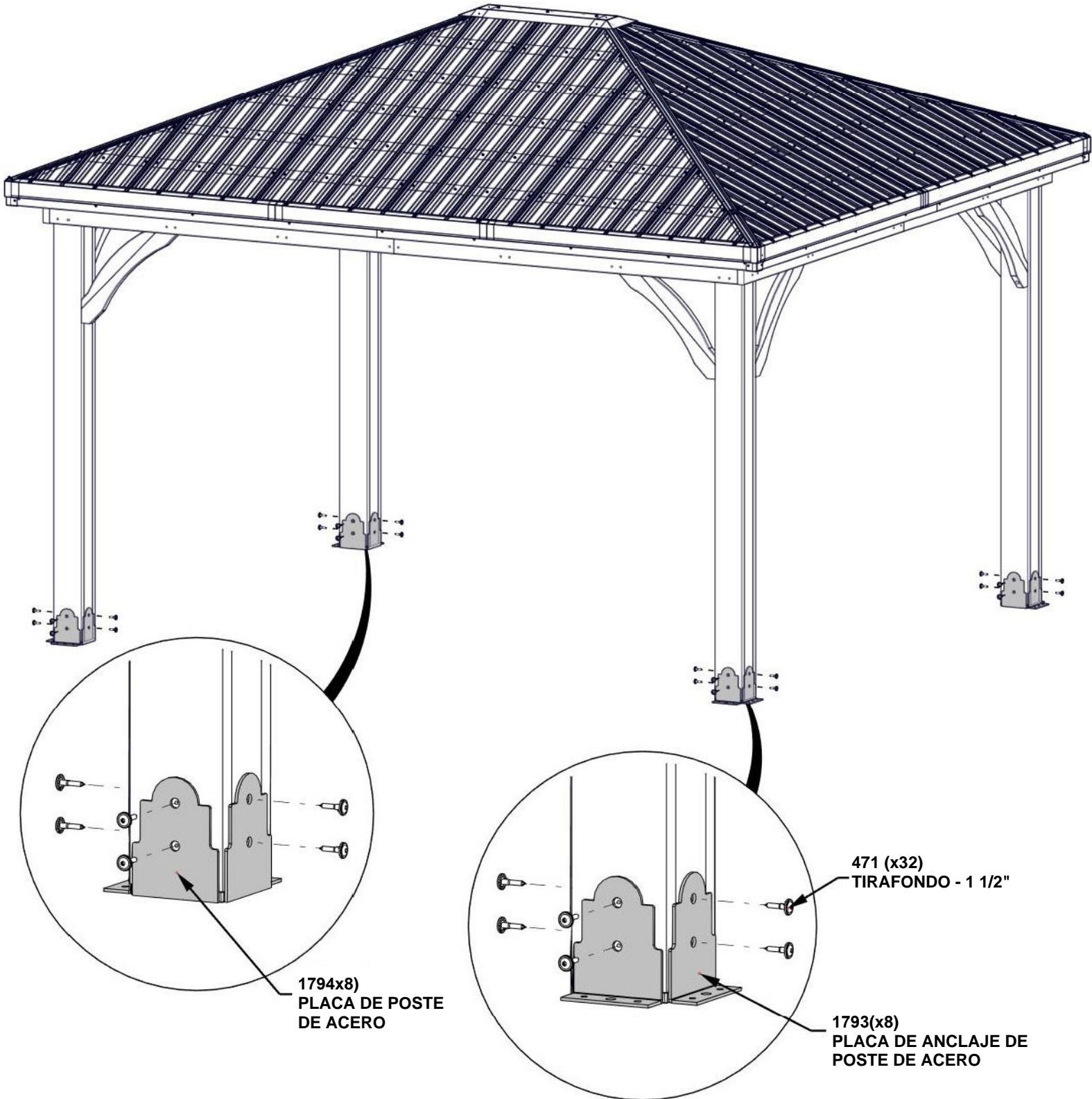
A4M01793 | PLACA DE ANCLAJE DE POSTE DE ACERO (8)
