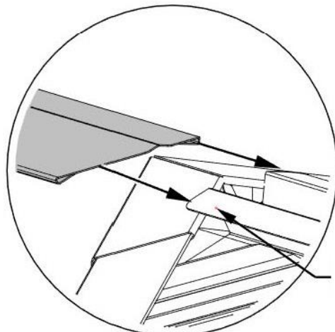
1258(x1) MONTAJE DE EMPALME DE LA TAPA DE LA CUMBRERA
