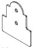
A4M01794 | PLACA DE POSTE DE ACERO (8)
