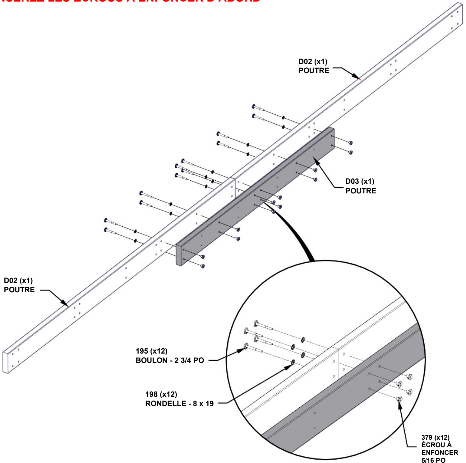
D02 | POUTRE - W4L15284 (2) | 1 3/8 po x 5 1/4 po x 59 1/16 po (36x134x2261)
