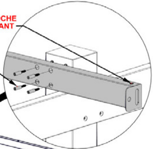
1103 (x4) VIS À SIX PANS CREUX TORX 1/4-20
