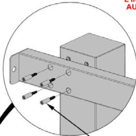
1103 (x4) VIS À SIX PANS CREUX TORX 1/4-20
