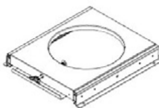
A13 MONTAGE DE HAUSSE DE BONBONNE DE GAZ - A4M03047 (x1) 1 15/16"x12 7/8"x14 3/4" (49x327x374)
