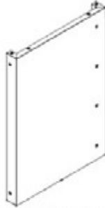
G7 MONTAGE DU MUR LATÉRAL D'ARMOIRE DROIT- A4M03041 (x1) 2 9/16"x23 3/8"x33 3/8" (65x594x848)
