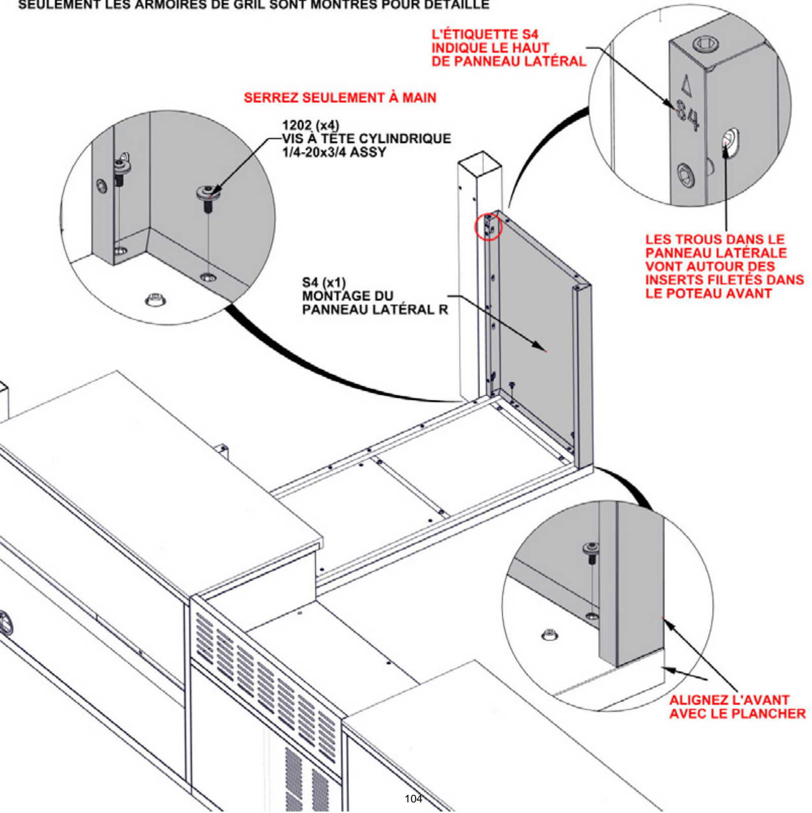
S4 MONTAGE DU PANNEAU LATÉRAL- A4M03093 (x1) 2 5/8"x23 3/8"x33 3/8" (67x594x848)
