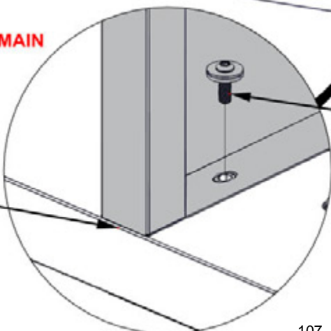
1202 (x2) VIS À TÊTE CYLINDRIQUE TORX 1/4-20x3/4 ASSY
