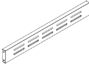
O8 PANNEAU DE VENTILATION DU FOUR À PIZZA - A4M03078 (x1) 1 3/16"x4"x31 7/16" (30x102x798)
