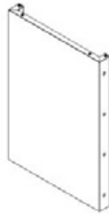
S4 MONTAGE DU PANNEAU LATÉRAL- A4M03093 (x1) 2 5/8"x23 3/8"x33 3/8" (67x594x848)
