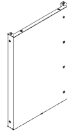
G7 MUR LATÉRAL DE L'ARMOIRE D'ANGLE DROIT - A4M03041 (x1) 2 9/16"x23 3/8"x33 3/8" (65x594x848)
