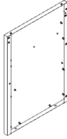
G6 MUR LATÉRAL DE L'ARMOIRE D'ANGLE DROIT - A4M03040 (x1) 2 1/16"x23 3/8"x33 3/8" (53x594x848)
