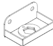
A9 SUPPORT DU TUYAU D'ARROSEMENT - A4M03060 (x2) 1 1/4"x1 7/16"x2 9/16" (31.5x36.5x65)
