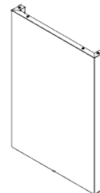
O5 ASSEMBLAGE DU PANNEAU LATÉRAL DE L'ARMOIRE DU FOUR À PIZZA - A4M03063 (x1) 2 5/8"x23 3/8"x33 3/8" (67x594x848)
