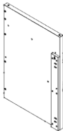
O2 ASSEMBLAGE DU PANNEAU LATÉRAL DE L'ARMOIRE DU FOUR À PIZZA - A4M03067 (x1) 2 5/8"x23 3/8"x33 3/8" (67x594x848)
