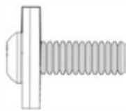
H101202 ENSEMBLE TÊTE PORTE-PLATEAU TORX (x120) 1/4-20x3/4"
