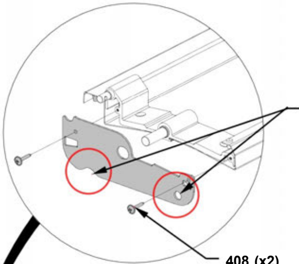
408 (x2) VIS -1/2"
