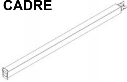
P02 POSTE -A4M01984 4 5/16"x6 (x1) 3/4"x99F 1/2" (110x172x2527)
