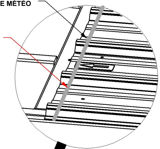
556 (x2) BANDE MÉTÉO
