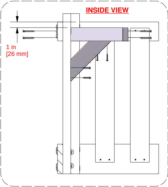
A4M02635 METAL ANGLE BRACE (x1)
