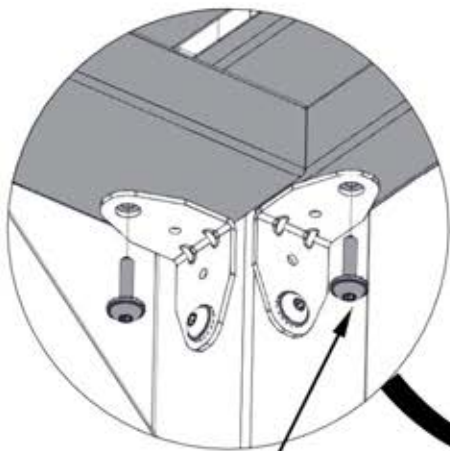
460 (x2) LAG SCREW - 1"
