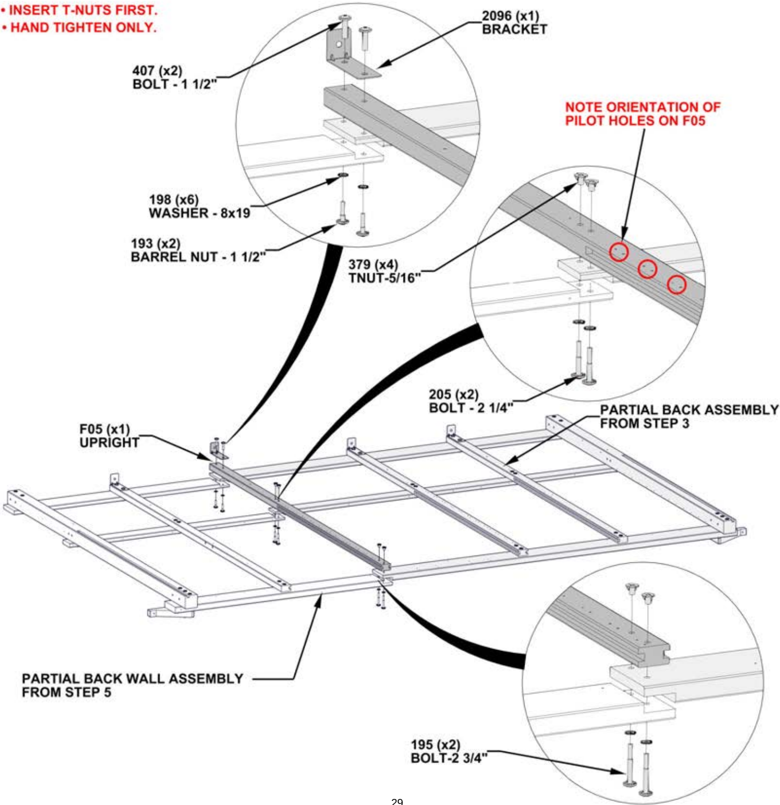
A4M02096 BRACKET (x1)
