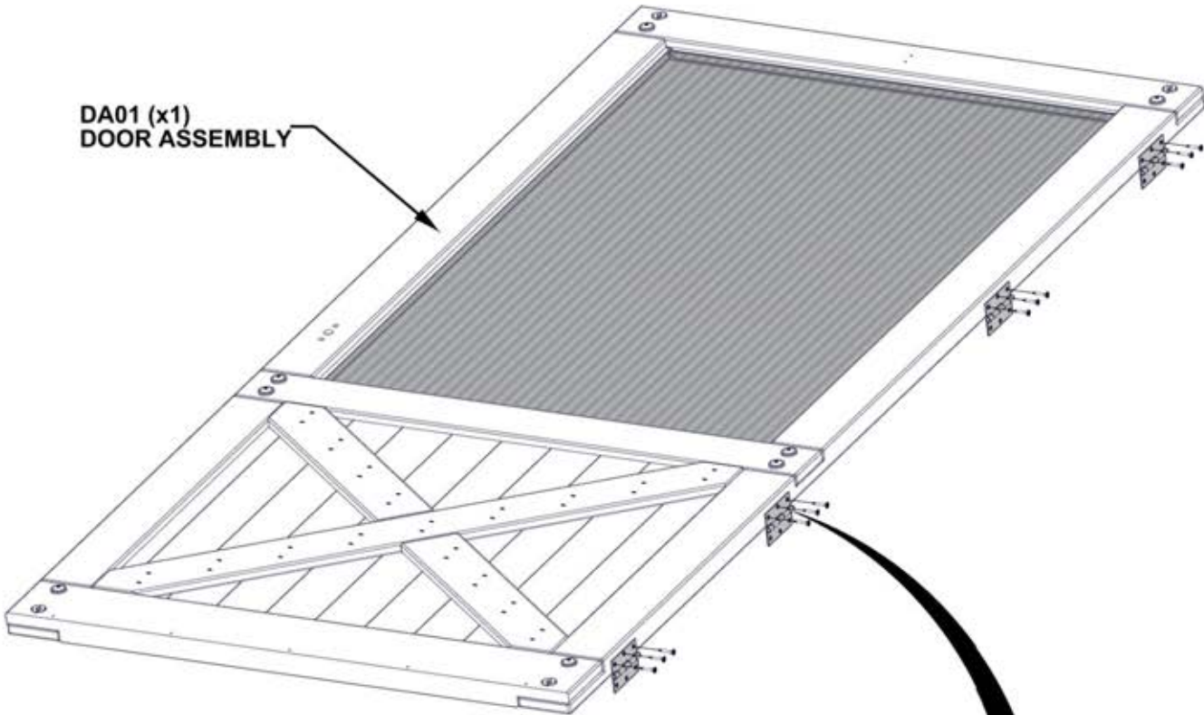
0557 (x4) HINGE
