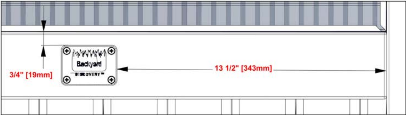
A4M02158 BYD ID TAG PATIO (x1)
