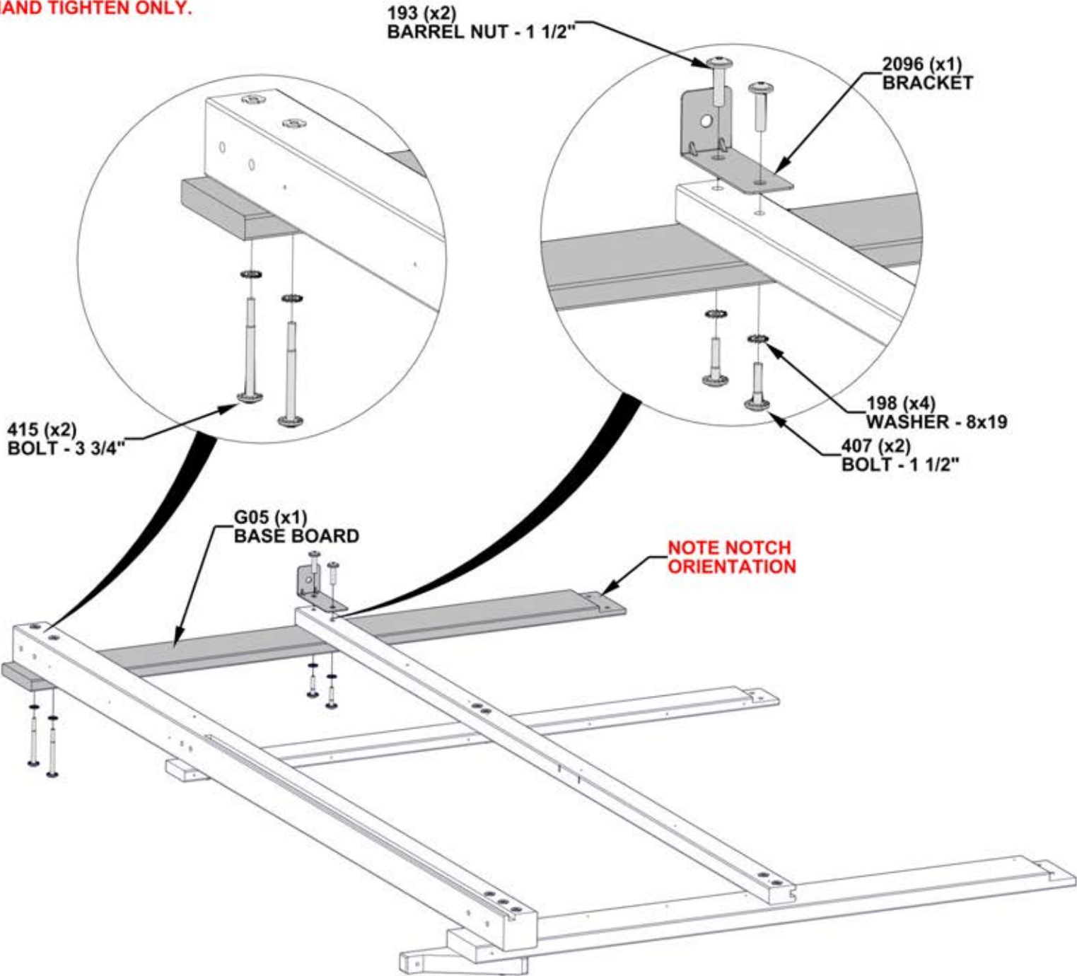
A4M02096 BRACKET (x1)
