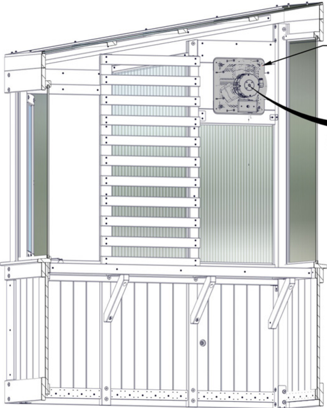
3475 (x1) EXHAUST FAN
