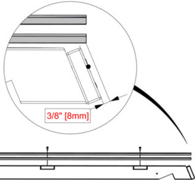
A4M02801 29GA STEEL SHEETING (x1)
