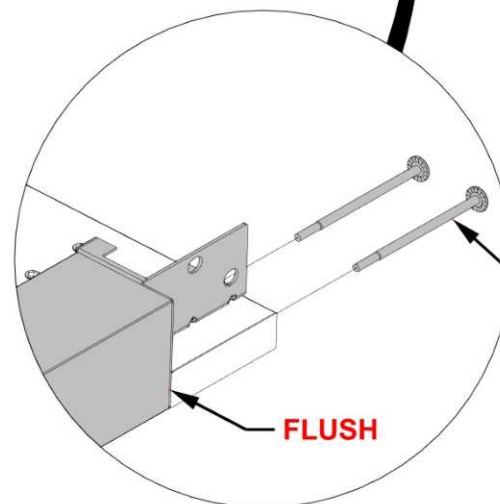
1230 (x2) BOLT - 6"
