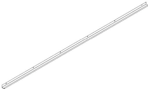
G01 CANALÓN - A4M01993 (x2) 1 9/16"x1 15/16"x108 7/8" (40x50x2765)
