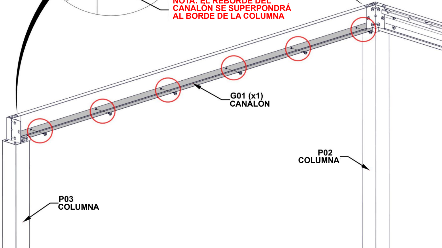
1202 (x6) TORNILLO TORX DE CABEZA PLANA 1/4-20x3/4" MONT
