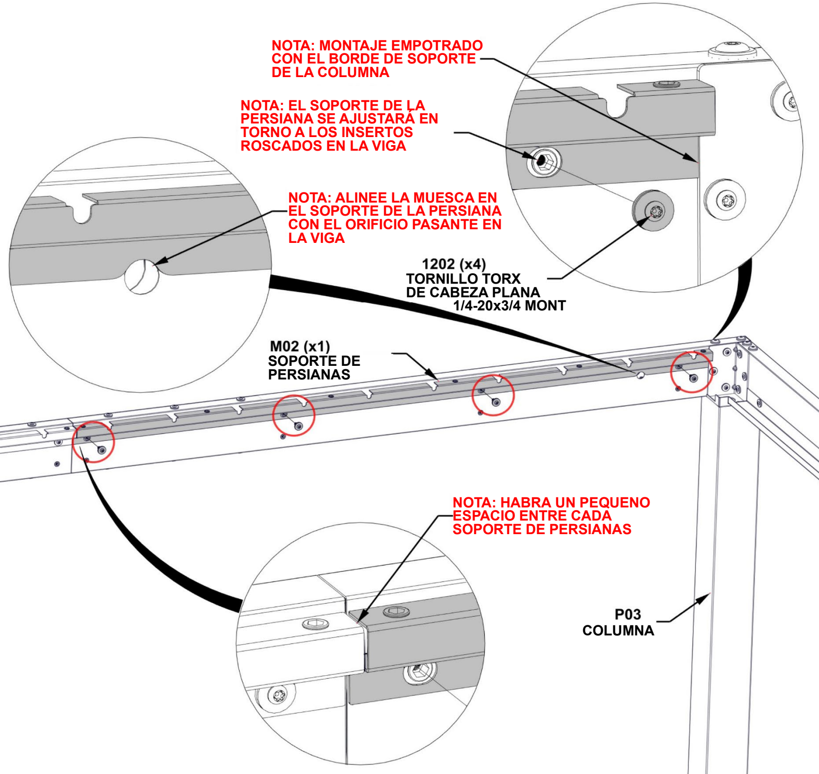
M02 SOPORTE DE PERSIANAS - A4M02865 (x1) 1"x1 15/16"x65 7/8" (25x49x1673)
