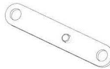
F03 CORREA DE ENLACE - A4M02229 (x1) 1/2"x11/16"x3 13/16" (13x17x97)
