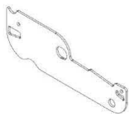
L02 PLACA LATERAL DE ACCIONAMIENTO DE LA (x1) PERSIANA- A4M04139 1/16"x2 3/16"x6 9/16" (2x55x167)
