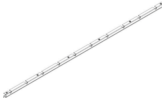
M01 SOPORTE DE LAS PERSIANAS- A4M02864 (x2) 1"x1 15/16"x65 7/8" (25x49x1673)
