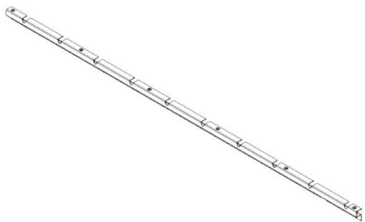
M02 SOPORTE DE PERSIANAS - A4M02865 (x1) 1"x1 15/16"x65 7/8" (25x49x1673)
