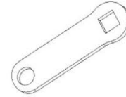
F04 CORREA DE ENLACE - A4M02225 (x1) 1/8"x13/16"x2 5/8" (3x20x66)
