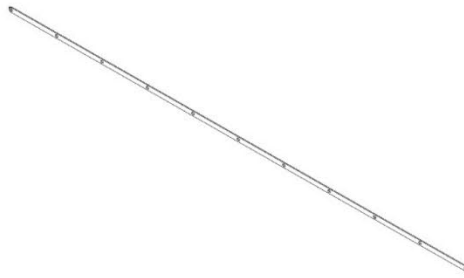
F02 CORREA DE SUJECIÓN PARA PERSIANAS - A4M02860 (x4) 1/8"x13/16"x68 1/16" (3x20x1730)
