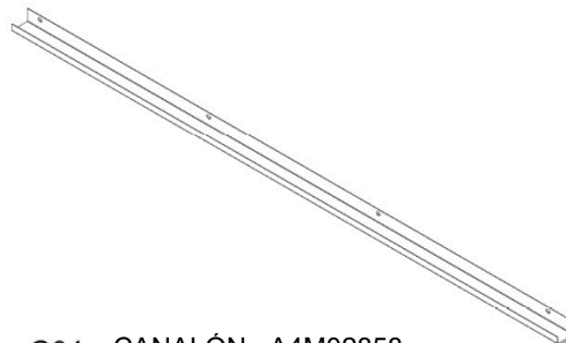
G04 CANALÓN - A4M02858 (x2) 1 9/16"x1 15/16"x65 15/16" (40x50x1675)
