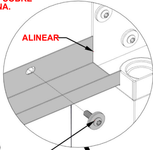
1202 (x6) TORNILLO TORX DE CABEZA PLANA 1/4-20x3/4" MONT
