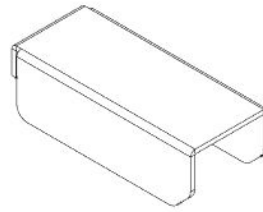
A5 SHELF BRACKET - A4M03141 (x8) 5/8"x7/8"x2 1/16" (16x22x53)
