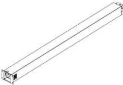
P03 POST - A4M05810 (x1) 5 1/2"x8"x89" (140x202x2262)
