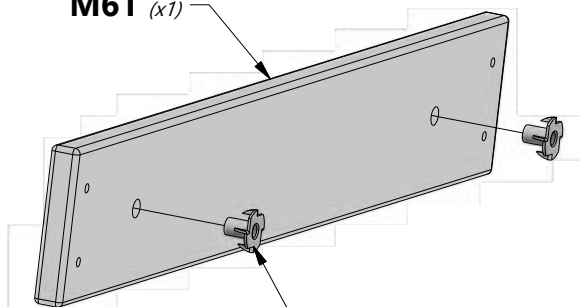
074 (x2) T-NUT - 5/16"
