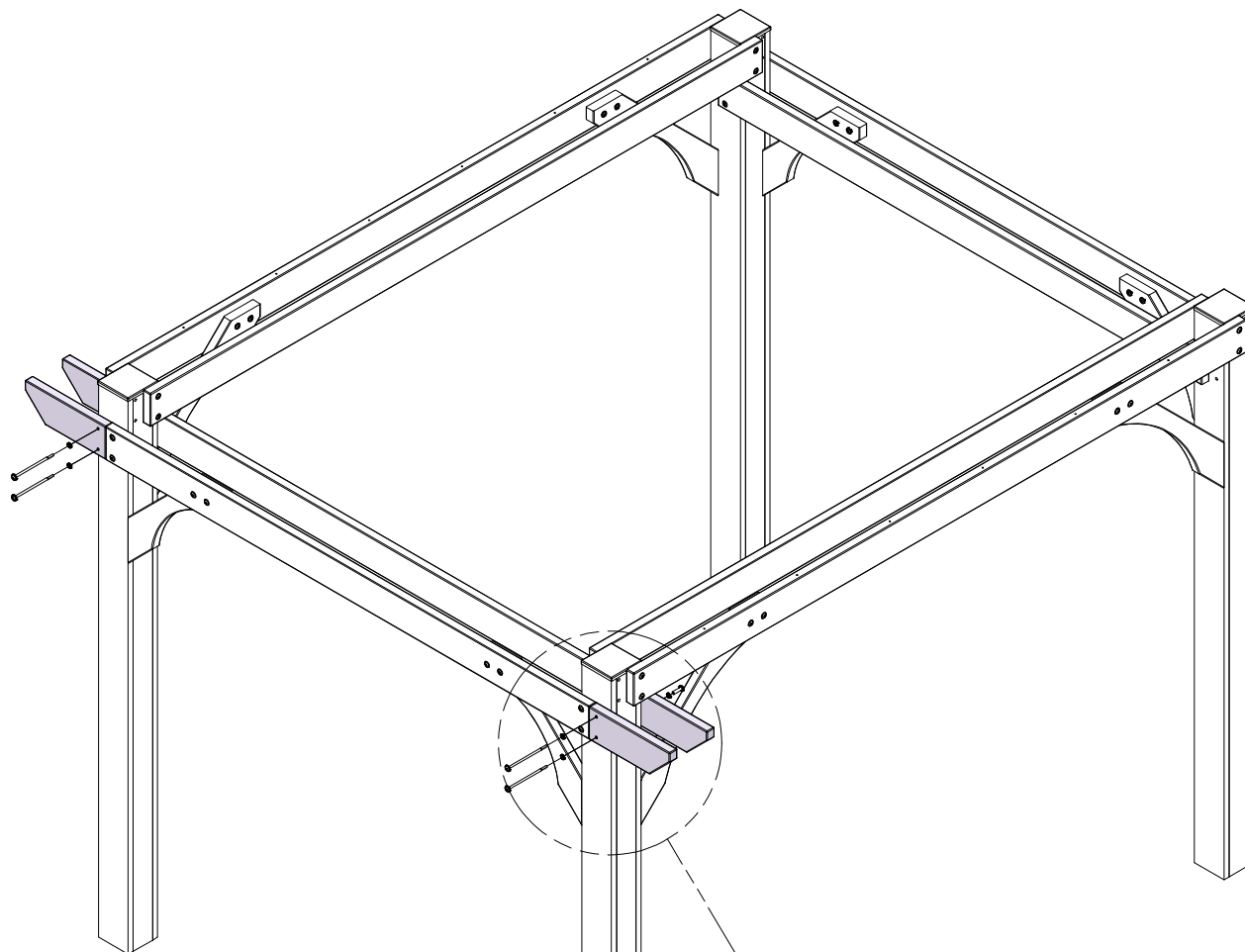
D6 EXTRÉMITÉ DE SOLIVE - W4L04588 (x4) 1 3/8"x5 1/4"x15" (36x134x381)
