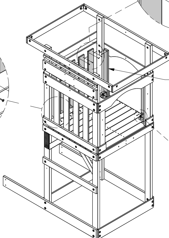
J1 (x2) WALL SLAT
