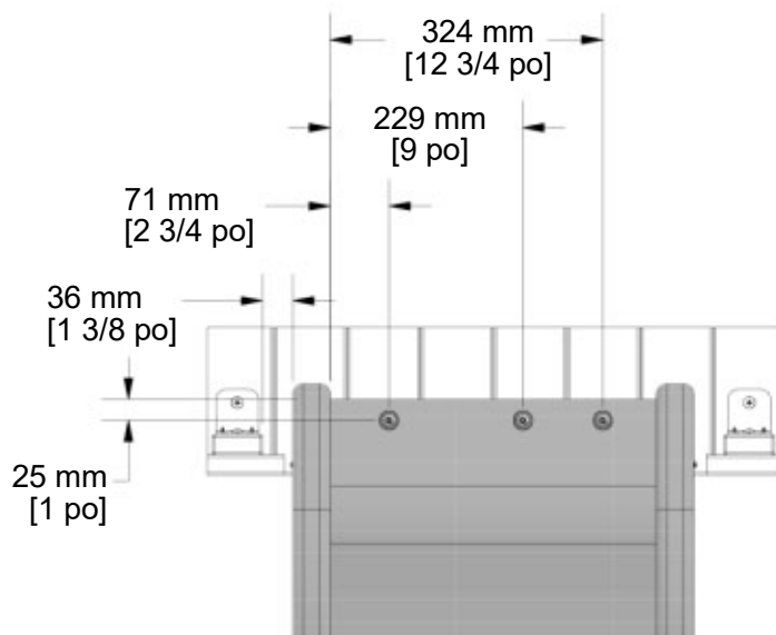
LIT DE TOBOGGAN CONGIFURATION DE PERÇAGE
