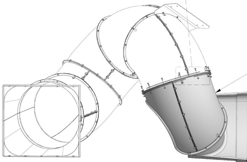
996 (x6) SUPPORT DE TOBOGGAN EN TUBE
